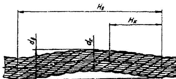
Рисунок 9. Волнистость каната
